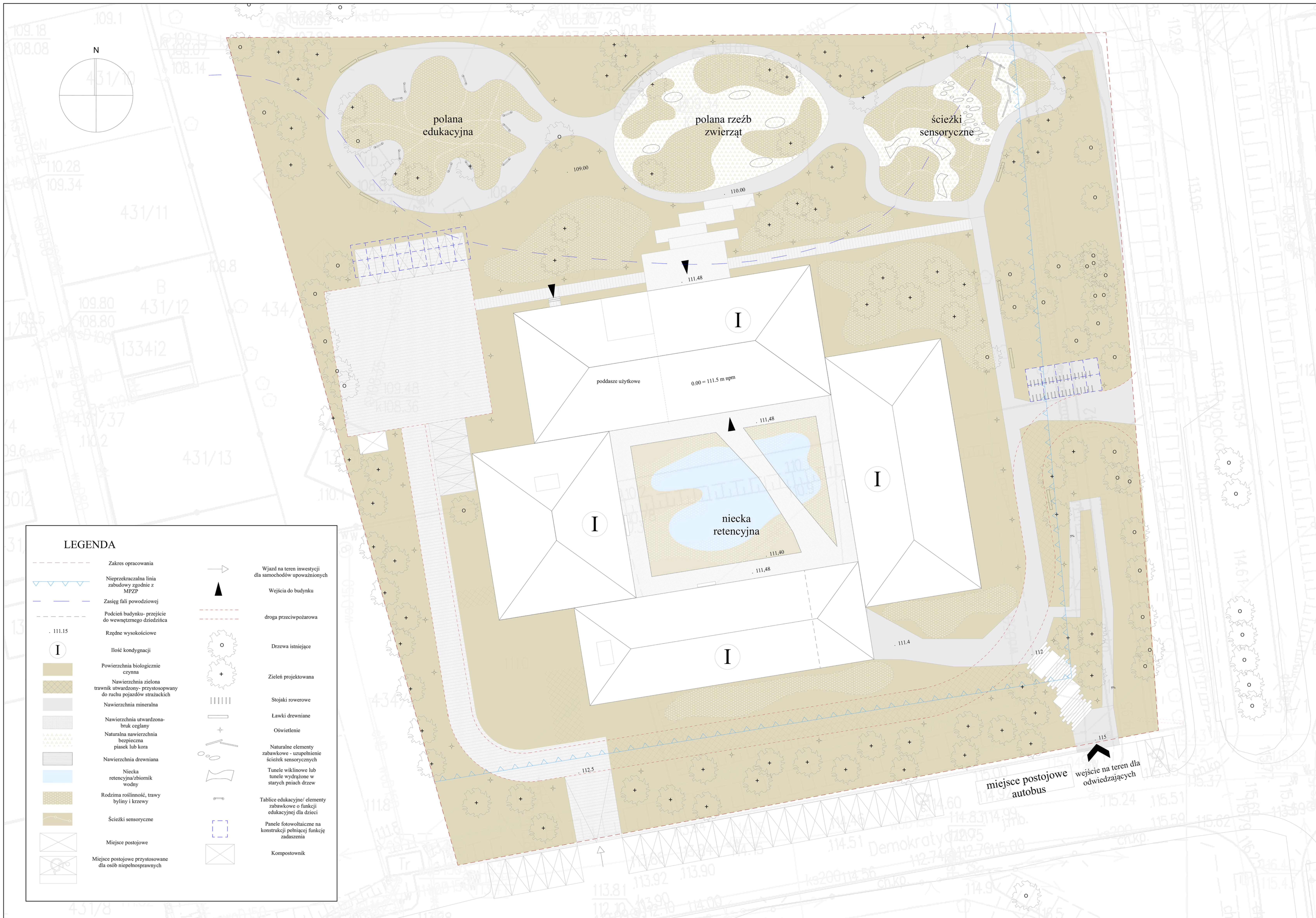
Koncepcja zagospodarowania terenu skala 1:200
